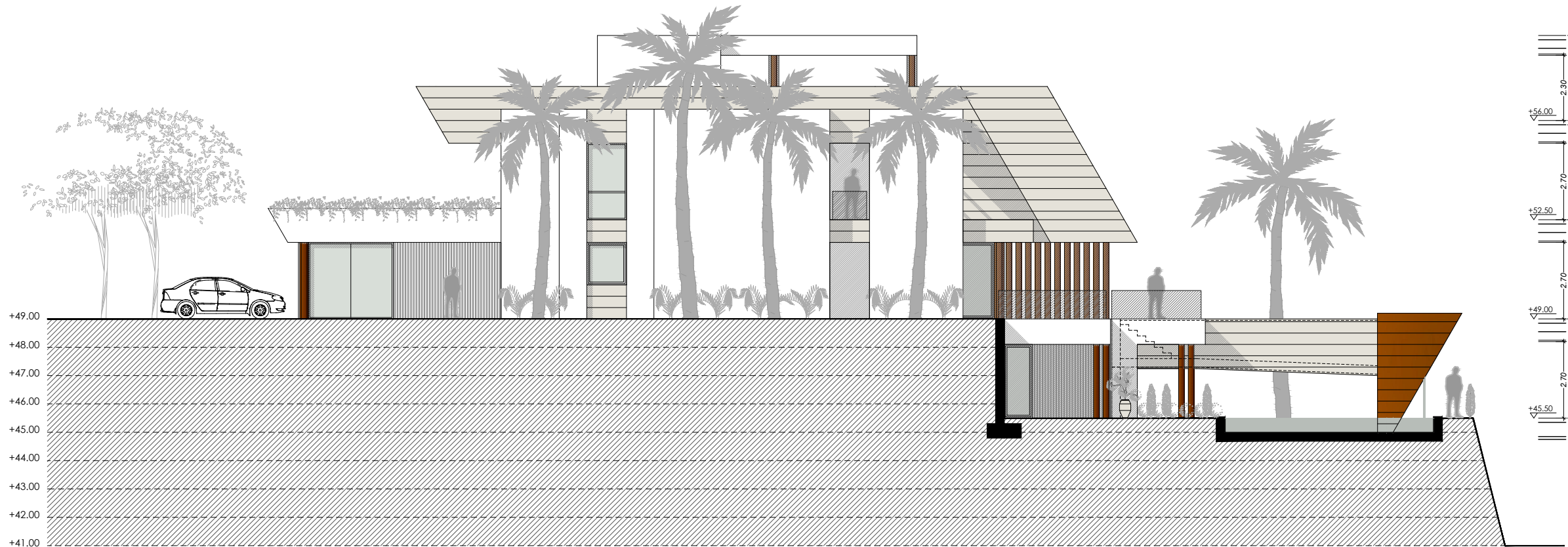
Alzado Suroeste
