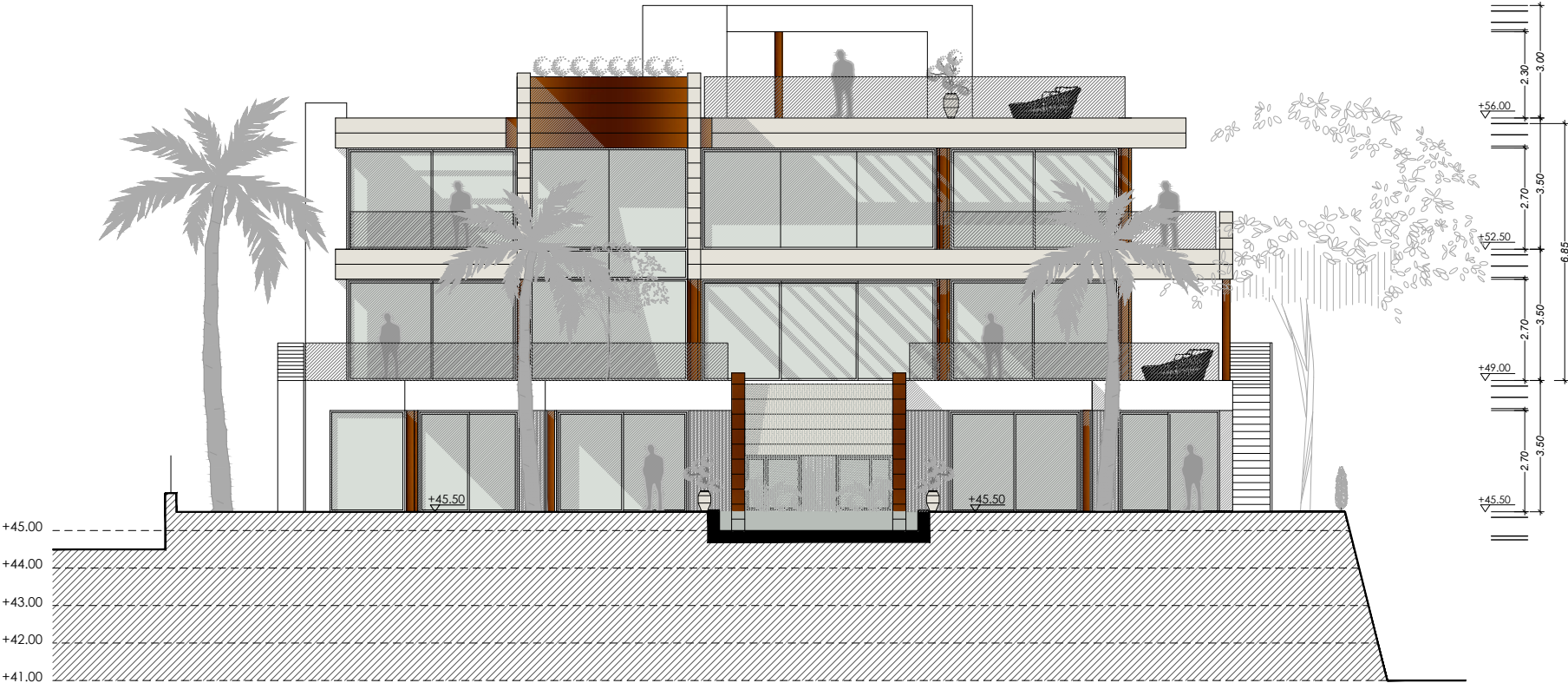
Alzado Sureste
